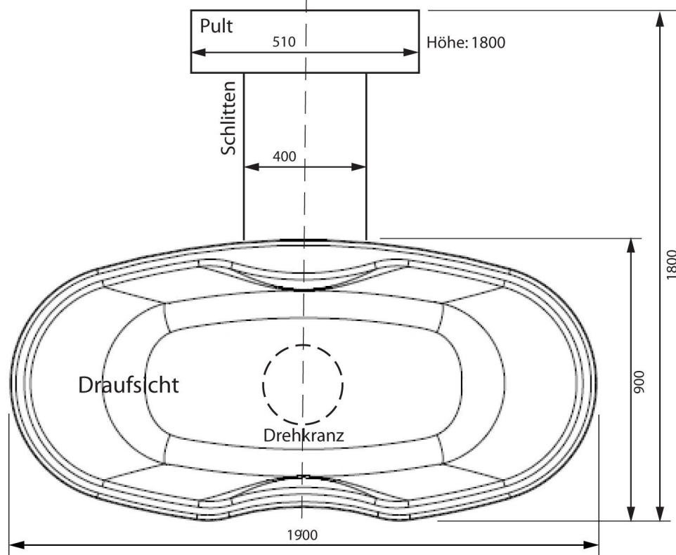
Ausgefahrene Position
